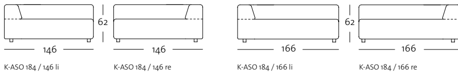
K-ASO 184 / 146 li
